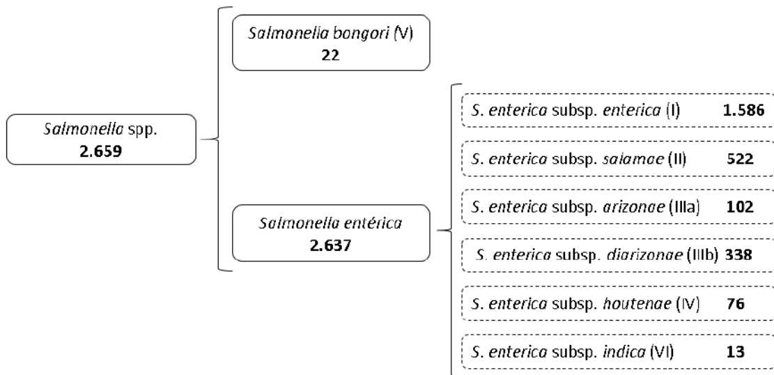
Figura 1. Esquema actual de la clasificación del género Salmonella * (Issenhuth-Jeanjean et al. , 2014).
