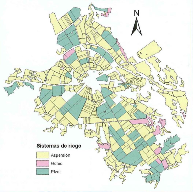
Figura 1. Plano parcelario de pivotes, coberturas fijas de aspersión y riego localizado en la Comunidad de Regantes de Candanos.
